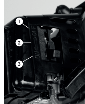
6 сурет. Ауа жапқышының иінтірегі
