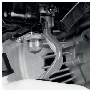
5 сур. Қолмен басқарылатын жанармай сорғысы
